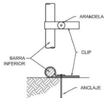
DETALLE ANCLAJES
