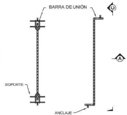
CANASTO INDIVIDUAL
