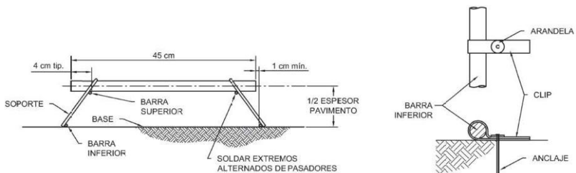
CORTE (B)
