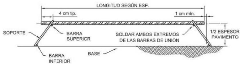
CORTE (B)
