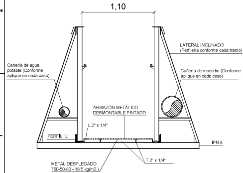
SECCIÓN TÍPICA
